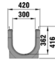
NW 300 Type 01
