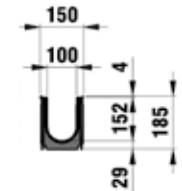
NW 100 Type 010
