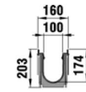
NW 100 Type 010
