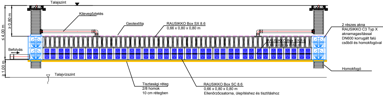
A-A metszet
