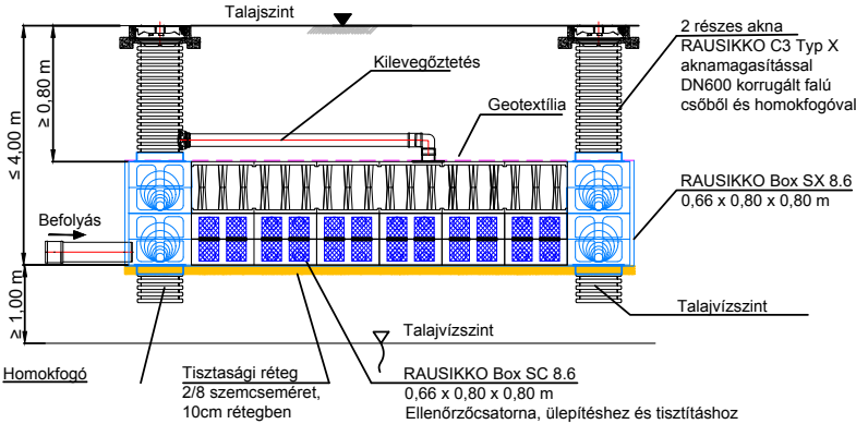
A-A metszet
